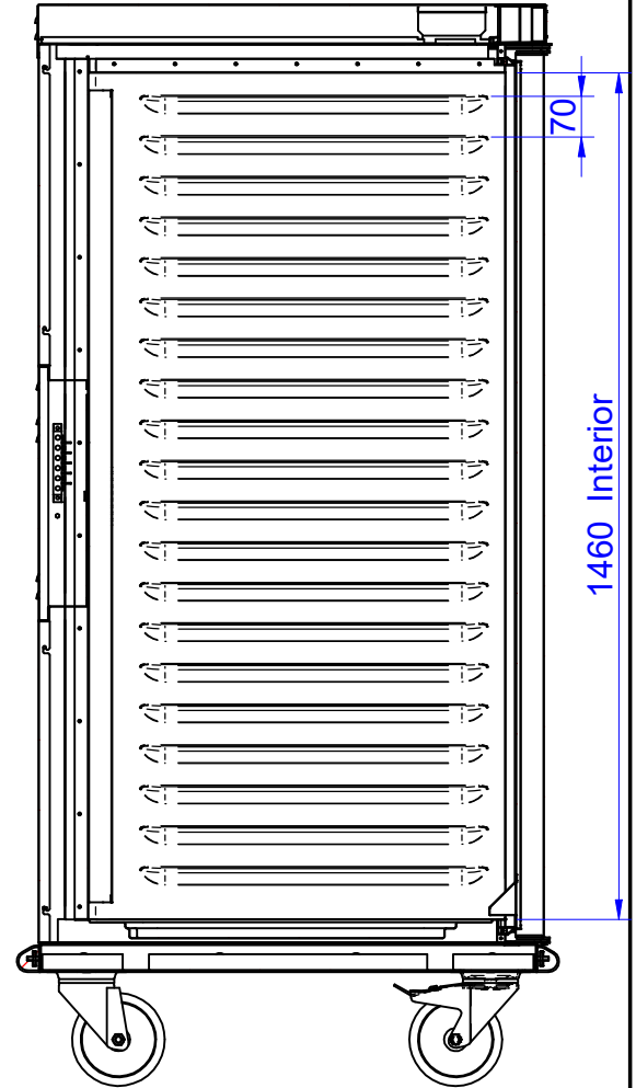
CORTE B-B
